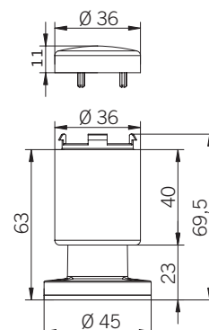
BASE CABLAGGIO WIRING BASE BASE DE CÂBLAGE
